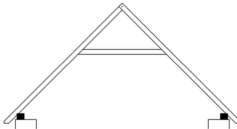
VAZNICOVÁ SOUSTAVA S HAMBALKEM
