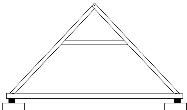
KROKEVNÍ SOUSTAVA S HAMBALKEM
